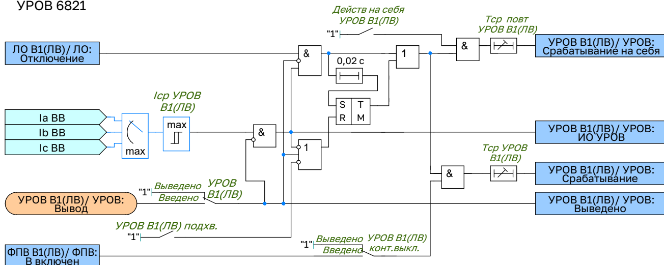
Рисунок 2.21 – Функциональная схема логики УРОВ
