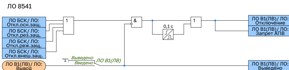
Рисунок 2.32 – Функциональная схема логики отключения В1(ЛВ)ВН
