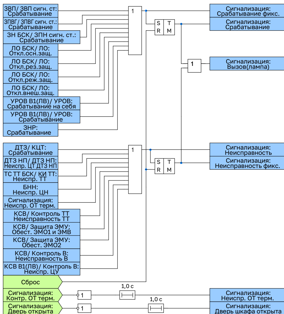
Рисунок 2.33 – Функциональная схема логики блока сигнализации
