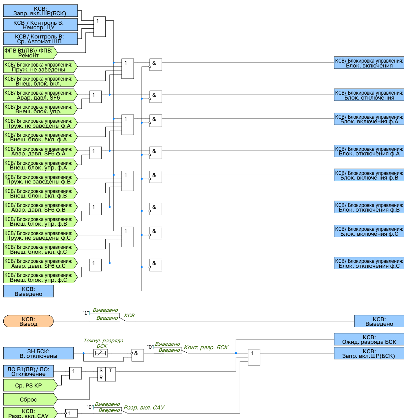
Рисунок 2.27 – Функциональная схема логики блокировки управления выключателя
